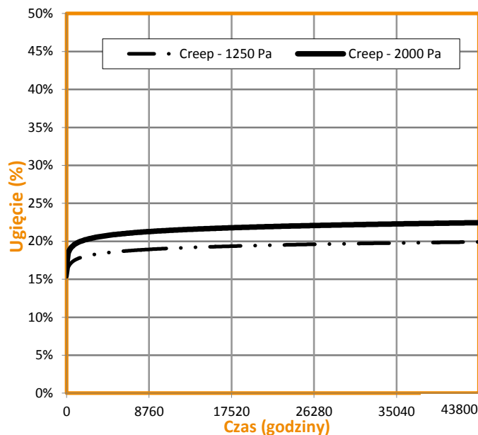
Pełzanie materiału - EN 1606 (4)
